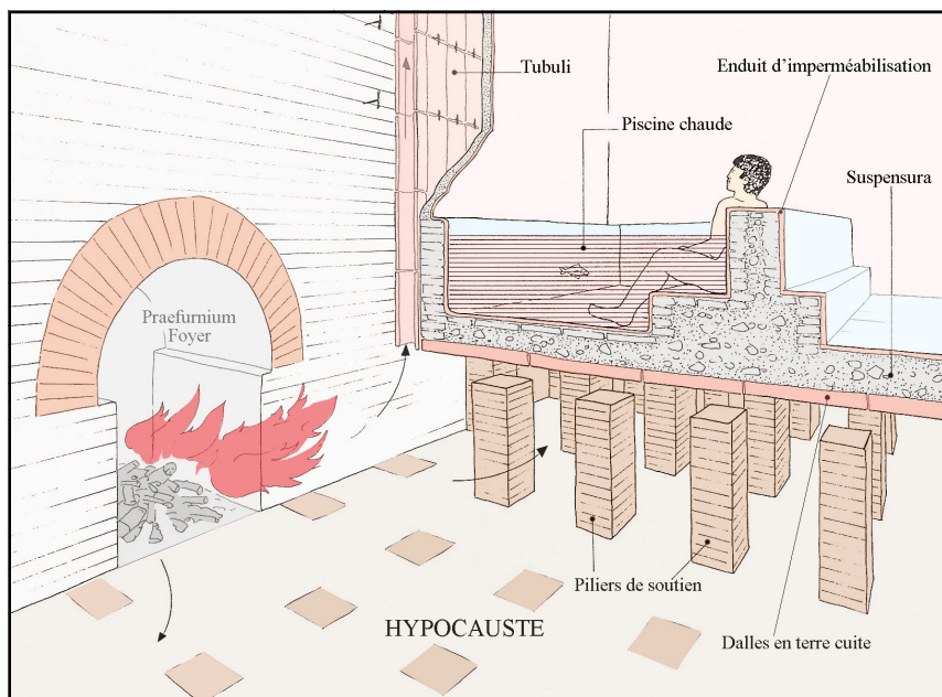
Le principe de l'hypocauste.
